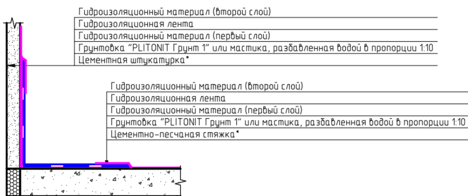
Разрез 1-1
