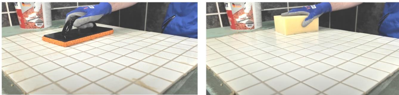
Рис. 36. Диагональными движениями шпателя убрать с поверхности плитки излишки затирки
